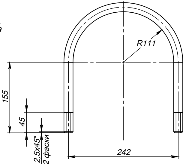
Поз.5 (Хомут)
