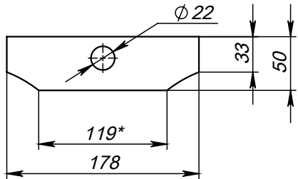
Поз.4 (Ушко) развертка
