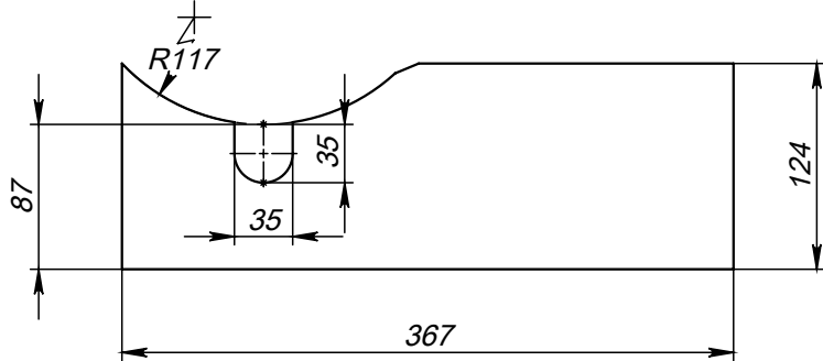
Поз.2 (Угольник) развертка
