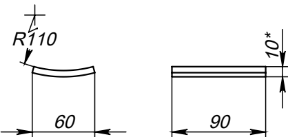
Поз.7 (Упор)
