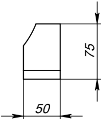
Поз.4 (Ушко)
